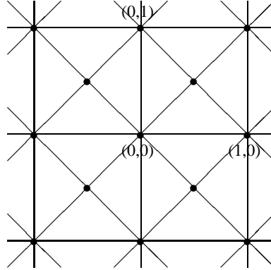
FIG. 2.1. Grid \Delta_0^{\mathbb{R}^2} .
